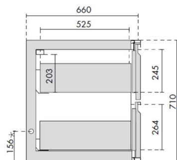
Ansicht Kühltisch mit Lade 1/2 - 1/2
