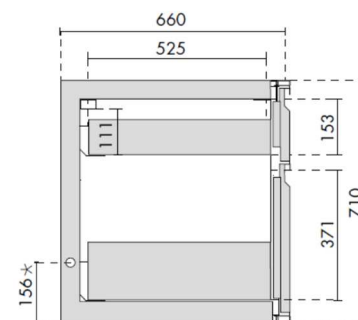
Ansicht Kühltisch mit Lade 1/3 - 2/3
