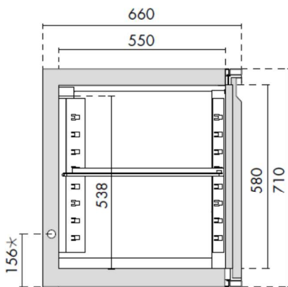
Ansicht Kühltisch mit Flügeltür
