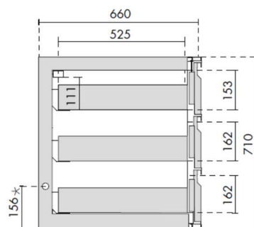
Ansicht Kühltisch mit Lade 1/3 - 1/3 - 1/3
