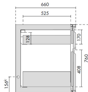
Ansicht Kühltisch mit Lade 1/3 - 2/3
