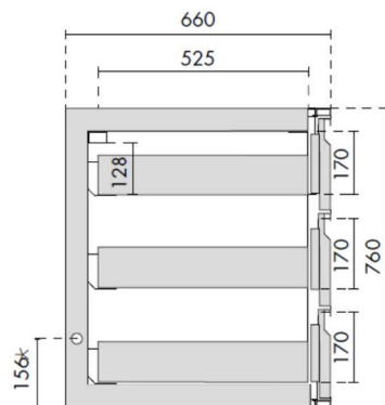
Ansicht Kühltisch mit Lade 1/3 - 1/3 - 1/3
