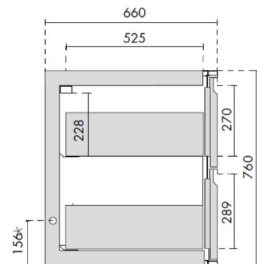
Ansicht Kühltisch mit Lade 1/2 - 1/2
