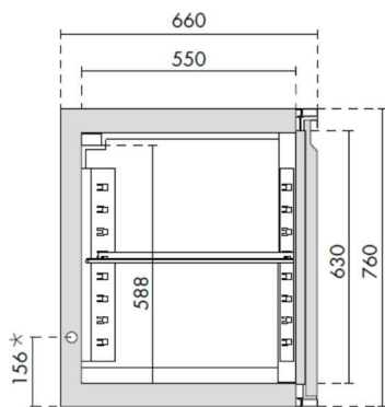
Ansicht Kühltisch mit Flügeltür
