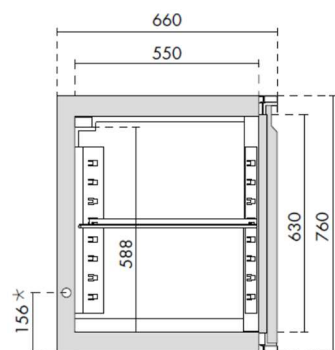
Ansicht Kühlpult mit Flügeltür
